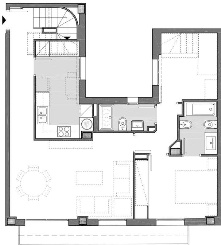
PLANTA INFERIOR
